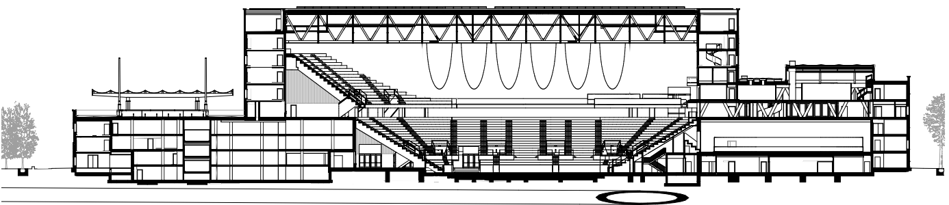
Längsschnitt
